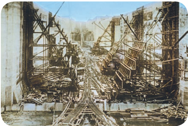
KANAŁ PANAMSKI - GÓRNE ŚLUZY W GATUN
